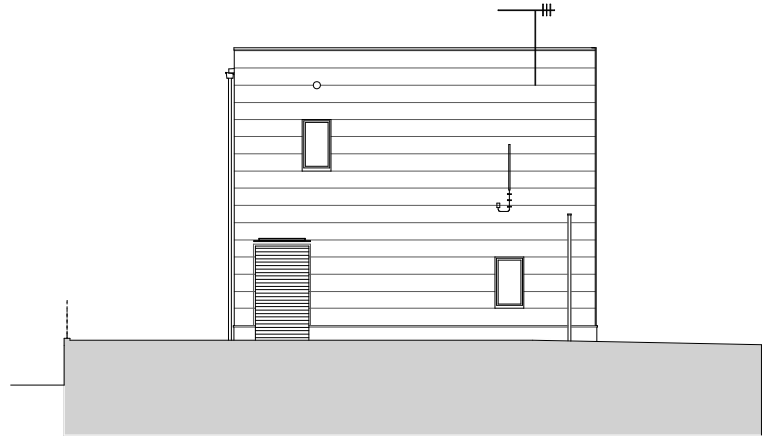
東立面図 1/200
