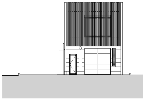
北立面図 1/200
