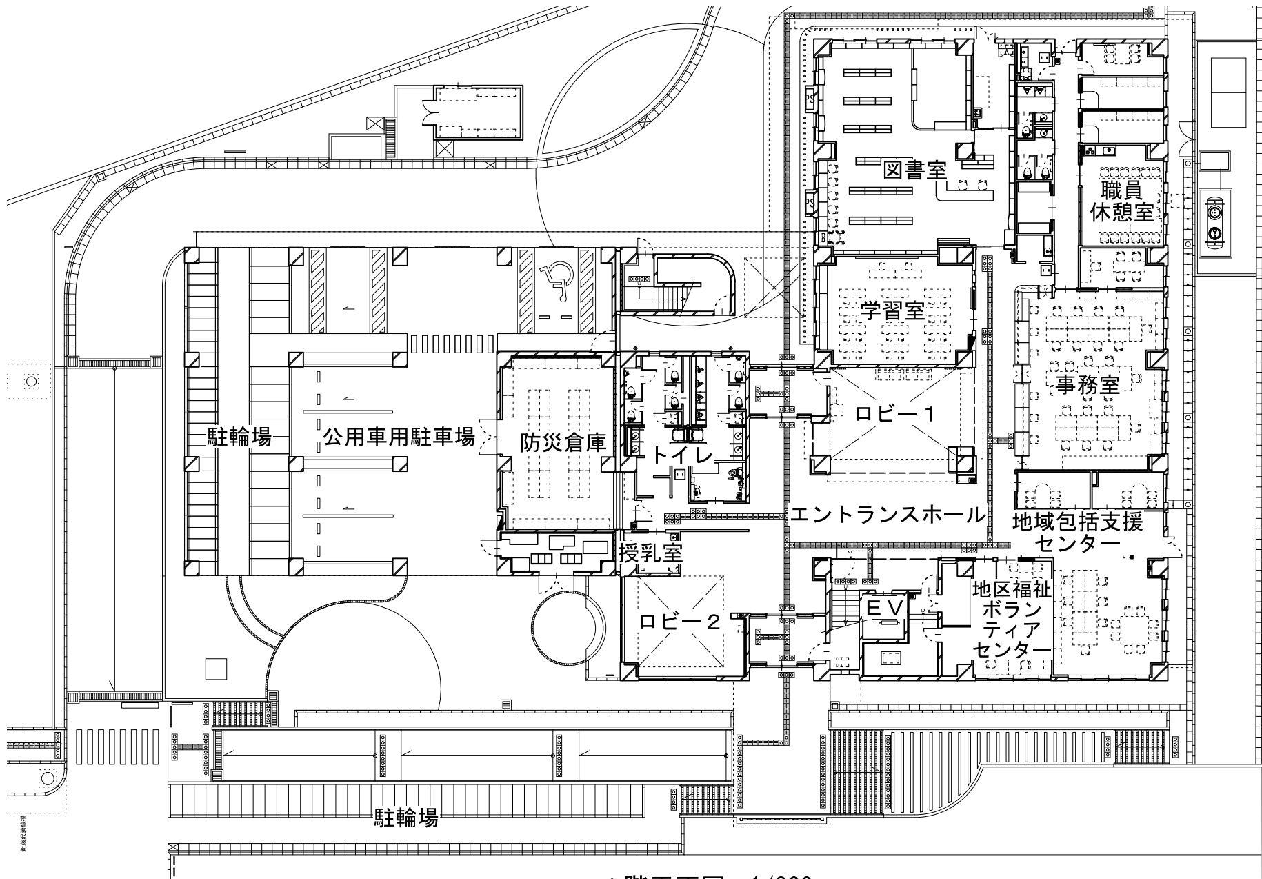
1階平面図 1/300
